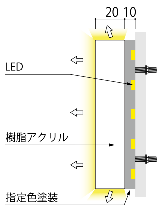
断面図 (単位:MM)
