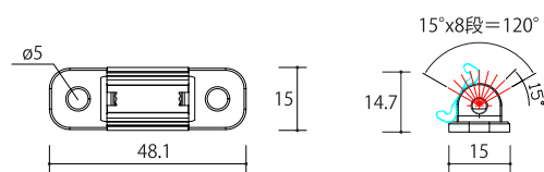
角度調整取付固定金具 (別売)
