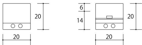
A-A断面図
