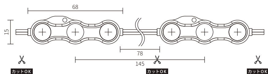
正面図 ※1個ごとにカット可能
